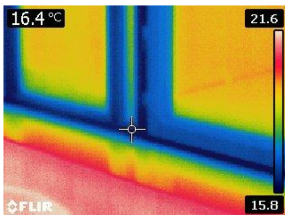
Figura 2.4 – Immagine termografica finestra
