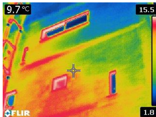
Figura 2.3 – Immagine termografica muro dall'esterno
